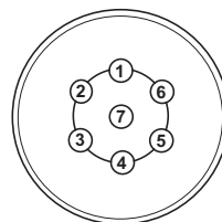
Connecture des câbles le jack à 7 poles
