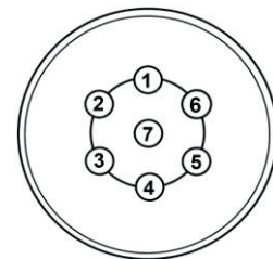
Tilslutning af ledninger i 7-polet forbindelsesdase
