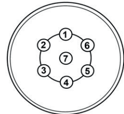
Podłączenie przewodów w gnieździe 7-biegunowym
