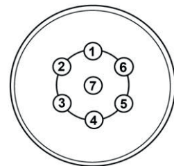
Collegamento dei cavi alla presa a 7 poli
