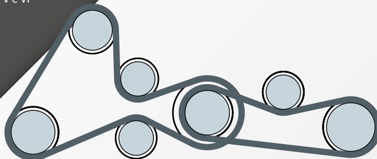
Fig 1 - Schema trasmissione ausiliaria (fino a codice motore n. 0113089 compreso), dotata di puleggia tendicinghia 37 93 0167 e cinghia Poly-V 37 92 8798
