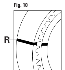
FIGURA 9 Insertar la herramienta específica de inmovilización de la polea de bomba de inyección "Q". FIGURA 10 Verificar la correcta alineación de las marcas de puesta a punto "R". FIGURA 11 Insertar las herramientas específicas para inmovilizar la polea de la bomba de inyección "S".
