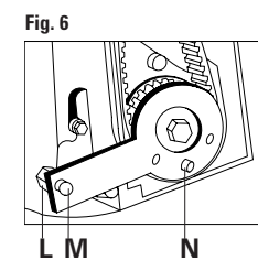
FIGURA 6 Desmontar el tornillo de la bomba de aceite L, y en su lugar, instalar el prisionero de la herramienta de inmovilización M. Rotar el cigüeñal hasta alcanzar el PMS del cilindro N° 1 y verificar la correcta posición de la marca de la polea del cigüeñal N. FIGURA 7 Insertar la herramienta especial de inmovilización del cigüeñal O. FIGURA 8 Insertar la herramienta específica para inmovilizar el volante motor P.
