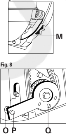
FIGURA 6 Insertar la herramienta específica para inmovilizar el volante motor M.
