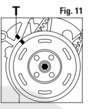
FIGURA 11 Verificar la correcta alineación de las marcas de fase T.
