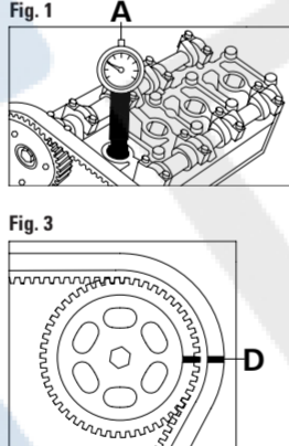
FIGURA 1 Insertar la herramienta comparadora A, sobre el cilindro N° 1.
