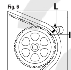
FIGURA 6 Controllare il corretto allineamento delle tacche di fase I con il bullone L.
