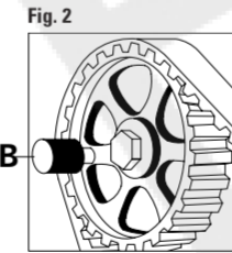
FIGURA 1 Controllare il corretto allineamento delle tacche di fase A. FIGURA 2 Inserire l'apposito attrezzo di bloccaggio dell'albero a camme B.
