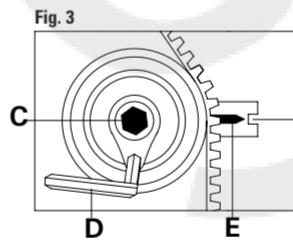
FIGURA 3 Allentare il bullone di bloccaggio C e ruotare in senso orario il tendicinghia, utilizzando la chiave esagonale D, fino ad allineare le tacche di fase E ed F; serrare quindi il bullone di bloccaggio C.
