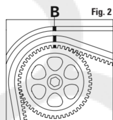
FIGURA 1 Controllare il corretto allineamento della tacca di fasatura, verificando che risulti allineata al carter distribuzione A. FIGURA 2 Controllare il corretto allineamento delle tacche di fase B.
