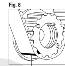
FIGURA 8 Controllare il corretto allineamento delle tacche di fase I.
