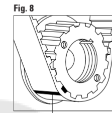
FIGURA 8 Verificar la correcta alineación de las marcas de puesta en fase I. FIGURA 9 Insertar la herramienta especial para inmovilización de cigüeñal motor L.
