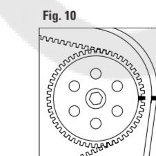
FIGURA 10 Controllare il corretto allineamento delle tacche di fase M (pompa Bosch).
