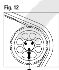
FIGURA 12 Insertar la herramienta para inmovilización de polea de bomba de inyeccion P. FIGURE 12 Introduire l'outil approprié de blocage poulie pompe d'injection P.
