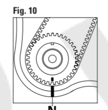
FIGURE 6 Introduire l'outil approprié de blocage vilebrequin G. FIGURE 7 Introduire l'outil approprié de blocage du volant H. FIGURE 8 Contrôler le correct alignement des points de repère de phase I. FIGURE 9 Contrôler le correct alignement des points de repère de phase L et introduire l'outil approprié de blocage vilebrequin M. FIGURE 10 Contrôler le correct alignement des points de repère de phase N. FIGURE 11 Introduire l'outil approprié de blocage du volant O.
