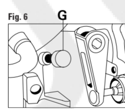
FIGURA 6 Insertar la herramienta especial para inmovilización de cigüeñal G. FIGURA 7 Insertar la herramienta de inmovilización del volante motor H.
