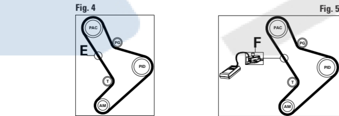
FIGURA 4 Punto de deflexión E. FIGURA 5 Insertar la herramienta apropiada para medición de la tensión de correa F en el punto indicado, y actuar sobre el tensor de la correa hasta conseguir un valor de tensión comprendido entre 88 y 122 Hz. FIGURE 2 Introduire l'outil approprié de réglage de tension B. FIGURE 3 Desserrer les boulons de blocage C et D du tendeur de courroie, En intervenant sur le tendeur de courroie dans sens des aiguilles de la montre, procéder jusqu'à la tension correcte appuyer un poids de 10kgs au point indiqué E, la courroie doit avoir une deflexion de 7-8mm, serrer ensuite les boulons de blocage C et D. FIGURE 4 Point de deflexion E. FIGURE 5 Introduire l'outil approprié de mesure de tension F, au point indiqué, et intervenir sur le tendeur de courroie jusqu'à atteindre une valeur comprise entre 88 et 112 Hz.
