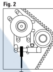
FIGURA 2 Insertar la herramienta apropiada para medición de la tensión de correa B. FIGURA 3 Aflojar los tornillos de ajuste C y D del tensor de la correa. Actuando sobre el tensor de la correa en sentido de las agujas del reloj, proceder hasta alcanzar la tensión correcta insertar un peso de 10 Kg en el punto indicado E. La correa debe tener un juego de aproximadamente 7 - 8 mm con respecto a su posición normal. Luego proceder al apriete de los tornillos de ajuste C y D.
