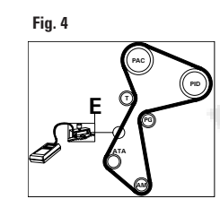
FIGURA 3 Allentare il bullone di bloccaggio C e inserire l'apposito attrezzo di tensionamento D, avvitandolo fino alla corretta tensione; serrare quindi il bullone di bloccaggio C. FIGURA 4 Inserire l'apposito attrezzo di misura del tensionamento E, nel punto indicato, ed agire sul tendicinghia fino ad un valore compreso tra 42,3 e 51,7 unità SEEM.
