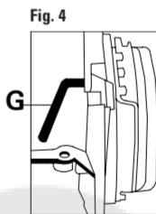
FIGURA 4 Insertar la herramienta de inmovilización del volante motor G. FIGURA 5 Insertar la herramienta específica para inmovilizar la correa de distribución H. FIGURA 6 Verificar la correcta alineación de las marcas de puesta en fase I.
