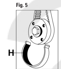
FIGURA 4 Insertar la herramienta de inmovilización del volante motor G. FIGURA 5 Insertar la herramienta específica para inmovilizar la correa de distribución H. FIGURA 6 Verificar la correcta alineación de las marcas de puesta en fase I.
