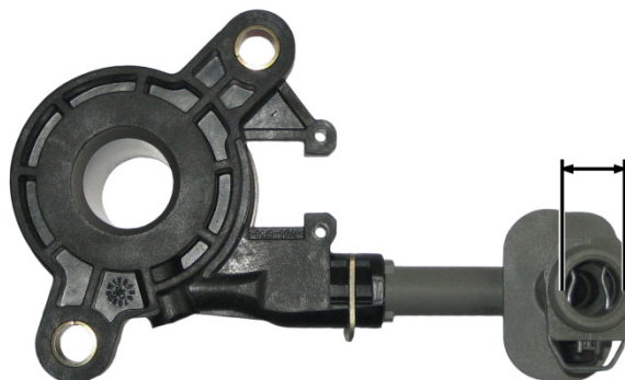
Kuva 2: CSC 3182 600 129 → 3182 654 146 → 3182 654 299 Hydrauliikkaliitännän halkaisija 13,3 mm
