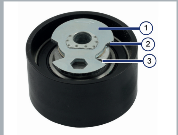
Bild 1: 55240 Halbautomatische Spannrolle
