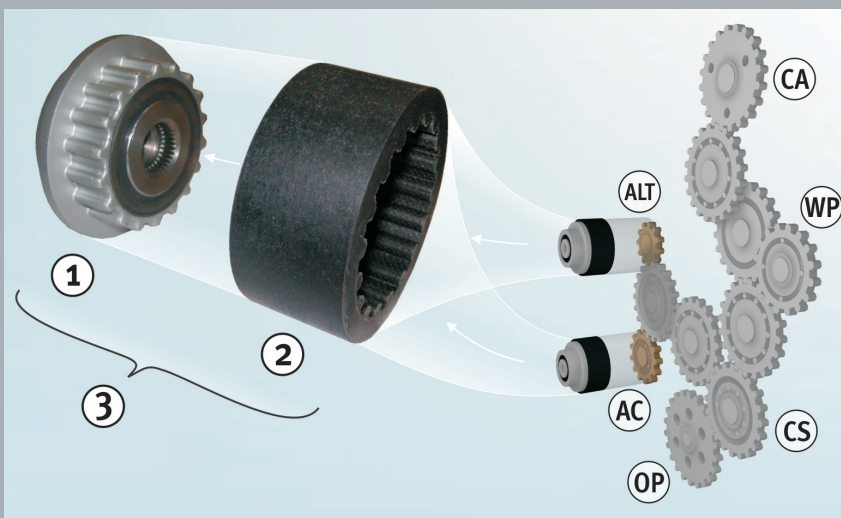
Bild 1: Generatorfreilauf mit flexibler Kupplungsmuffe und Stirnradtrieb
