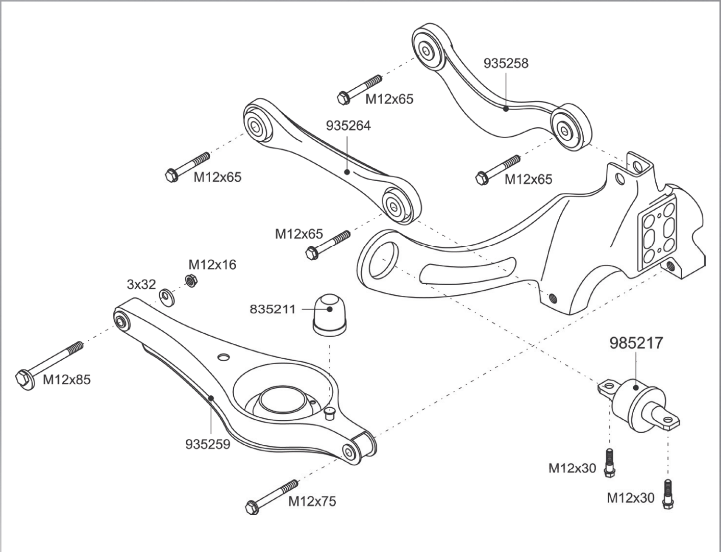
Илл. 1: фрагмент 935259S (рис.: левая сторона автомобиля)
