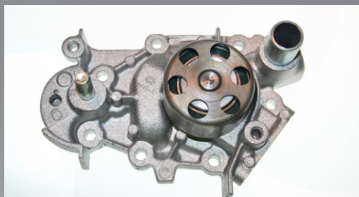
Bild 2: Neue Wasserpumpe 65569
