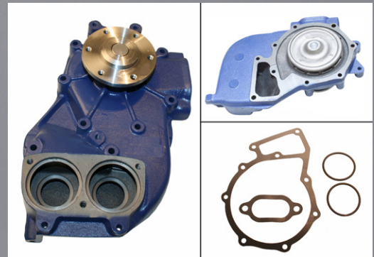
Bild 1: Wasserpumpe 65135 (ohne Thermostate)
