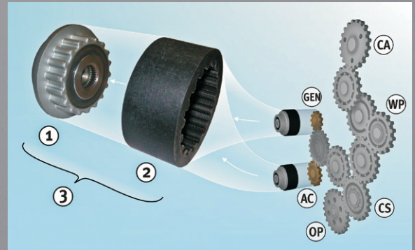
Bild 1: Generatorenfreilauf mit flexibler Kupplungsmuffe und Stirnradtrieb
