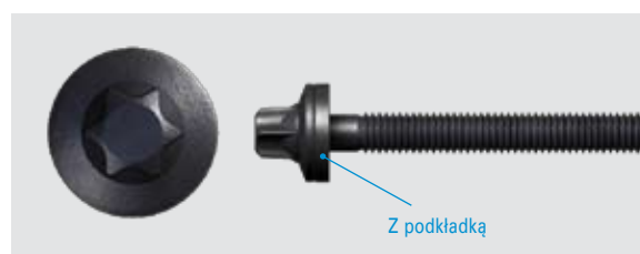
Rys. 1_Stara/zastąpiona śruba z podkładką (nr OE 607 926)
