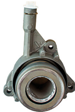
Afb. 2: Vorige CSC-versie 510 0092 10/11/12 met metalen drukring
