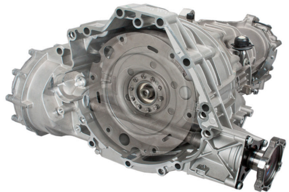
Εικόνα 1: Το εμπρόσθιο ημιαξόνιο περιστρέφεται μεταξύ του Βολάν Διπλής Μάζας (BDM) και της πλάκας εφαρμογής του.
