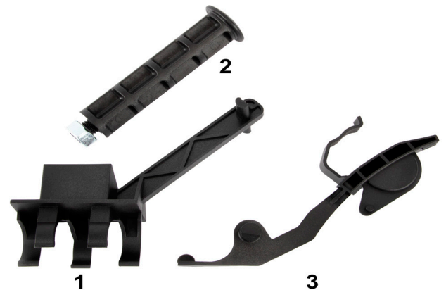
Εικόνα 2: Σετ ειδικών εργαλείων με Αρ. 400 0537 10
