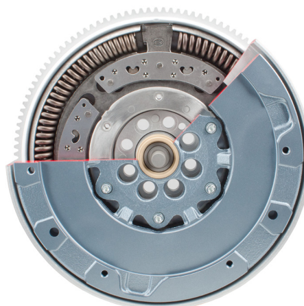
Bild 1: Dubbelmassesväghjul med centrifugalpendel i genomskärning
