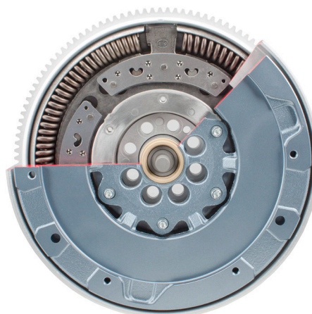
Рисунок 1: Двухмассовый маховик с демпфером маятникового типа
