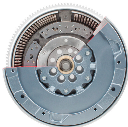
Fig. 1: Volant cu masă dublă, cu pendul pentru reducerea forței centrifuge
