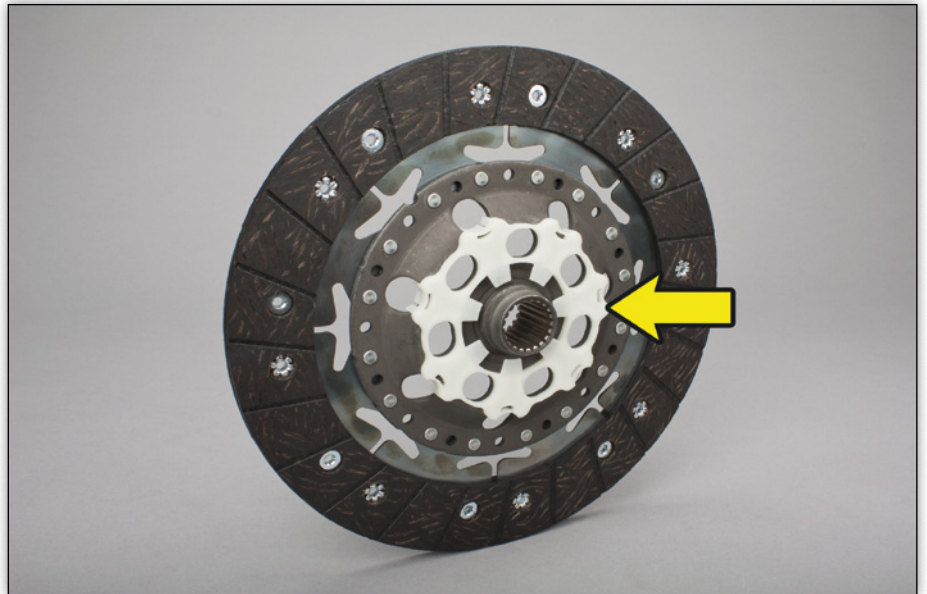
Fig. 1: LuK-koppelingsplaat met kunststof ring
