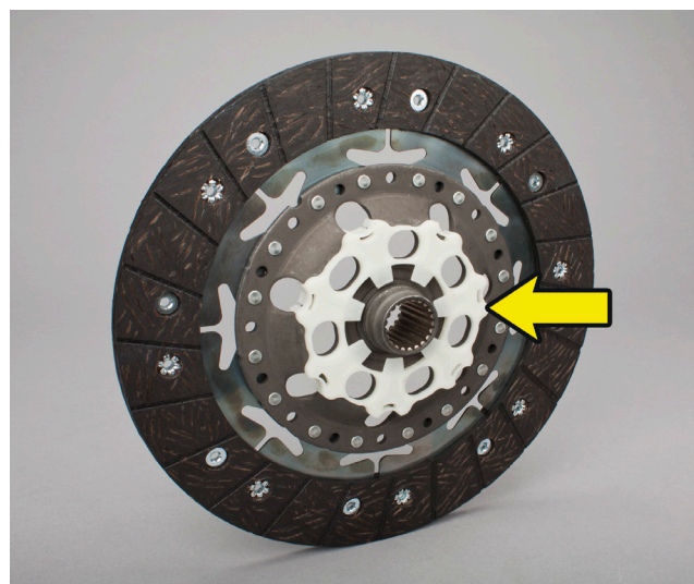
Billede 1: LuK koblingslamel med plastring
