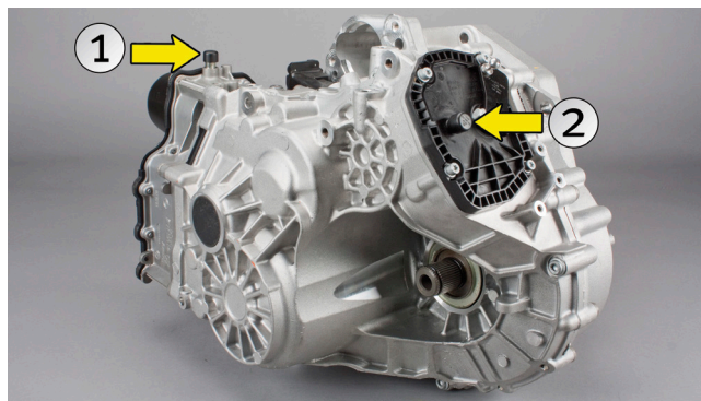
Fig. 1: Cutie de viteze automată cu capace de aerisire pentru unitatea mecatronică (1) și cutia de viteze (2).
