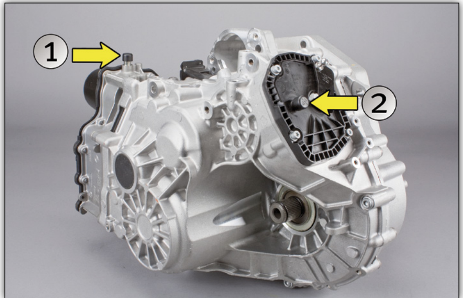
Fig. 1: DSG met ontluichtingsdoppen voor Mechatronic (1) en transmissie (2)
