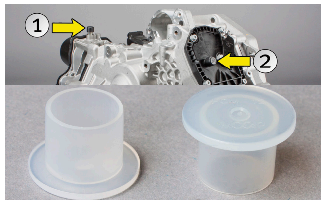
Εικόνα 2: Πάματα στεγανότητας
