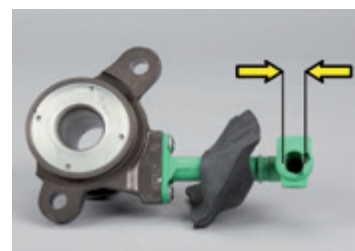
Fig. 4: LuK CSC 510 0137 10 Ligação hidráulica 12,2 mm
