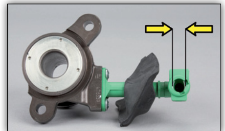
Fig. 4: LuK hydraulisch scharnierstuk 510 0137 10 hydraulische aansluiting 12,2 mm
