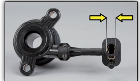
Fig. 2: LuK hydraulisch scharnierstuk 510 0097 10 hydraulische aansluiting 13,3 mm
