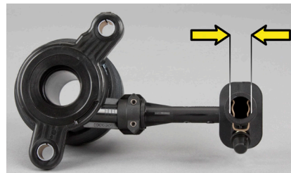
Εικόνα 2: Υδραυλικός σύνδεσμος 13.3 mm για το LuK CSC 510 0097 10
