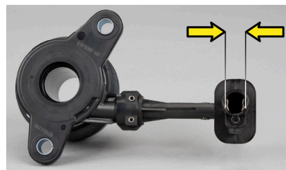
Εικόνα 1: Υδραυλικός σύνδεσμος 12.2 mm για το LuK CSC 510 0090
