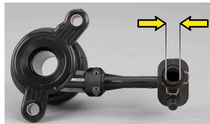
Εικόνα 3: Υδραυλικός σύνδεσμος 11.7 mm για το LuK CSC 510 0098 10
