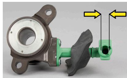
Εικόνα 4: Υδραυλικός σύνδεσμος 12.2 mm για το LuK CSC 510 0137 10
