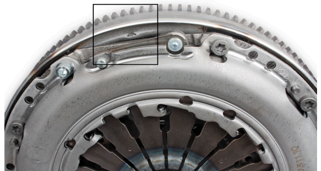
Зображення 1: пошкоджена деталь внаслідок застосування занадто довгих гвинтів
