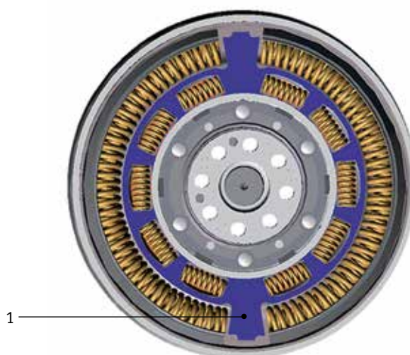
1 Äärik, millel on sisselõiked vedrude jaoks
