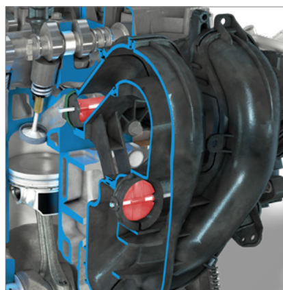
Válvulas en la tubería de aspiración
