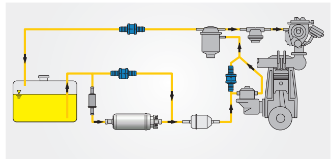
Esempio di impiego: Motore a carburazione con pompa supplementare elettrica inseribile
